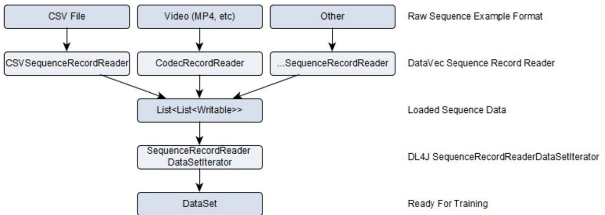
Figure F-2. DataVec sequence pipeline
